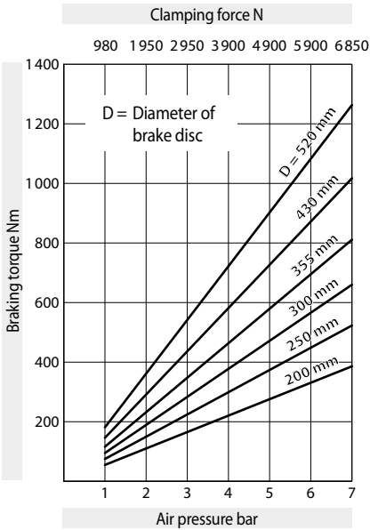
Brake Caliper DH 025 PFM - 635
