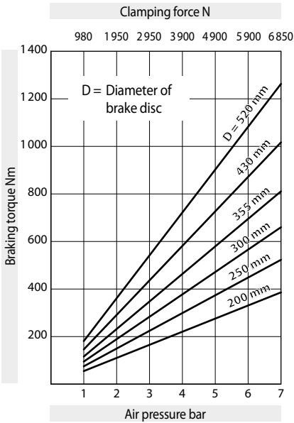
Brake Caliper DH 030 PFM - 635
