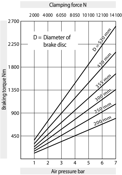
Brake Caliper DH 025 PFM - 655
