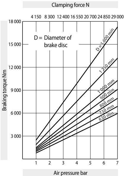
Brake Caliper DU 060 PFM - 660
