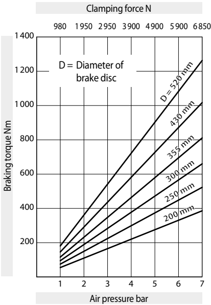
Brake Caliper DV 030 PFM - 635
