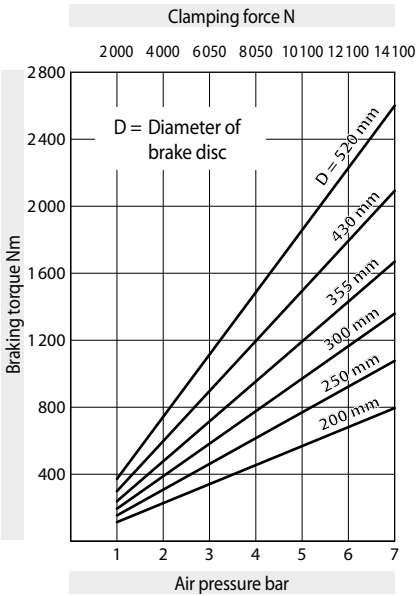
Brake Caliper DV 030 PFM - 655
