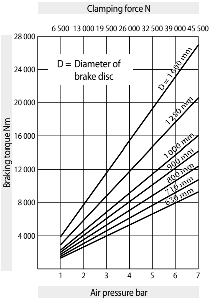
Brake Caliper DU 060 PFM - 680
