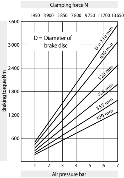
Brake Caliper DH 035 PFM - 655
